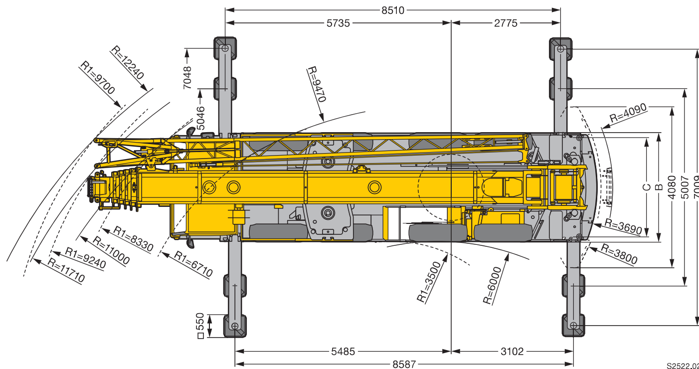
Maße · Dimensions · Encombrement · Dimensioni · Dimensiones · Размеры mm
